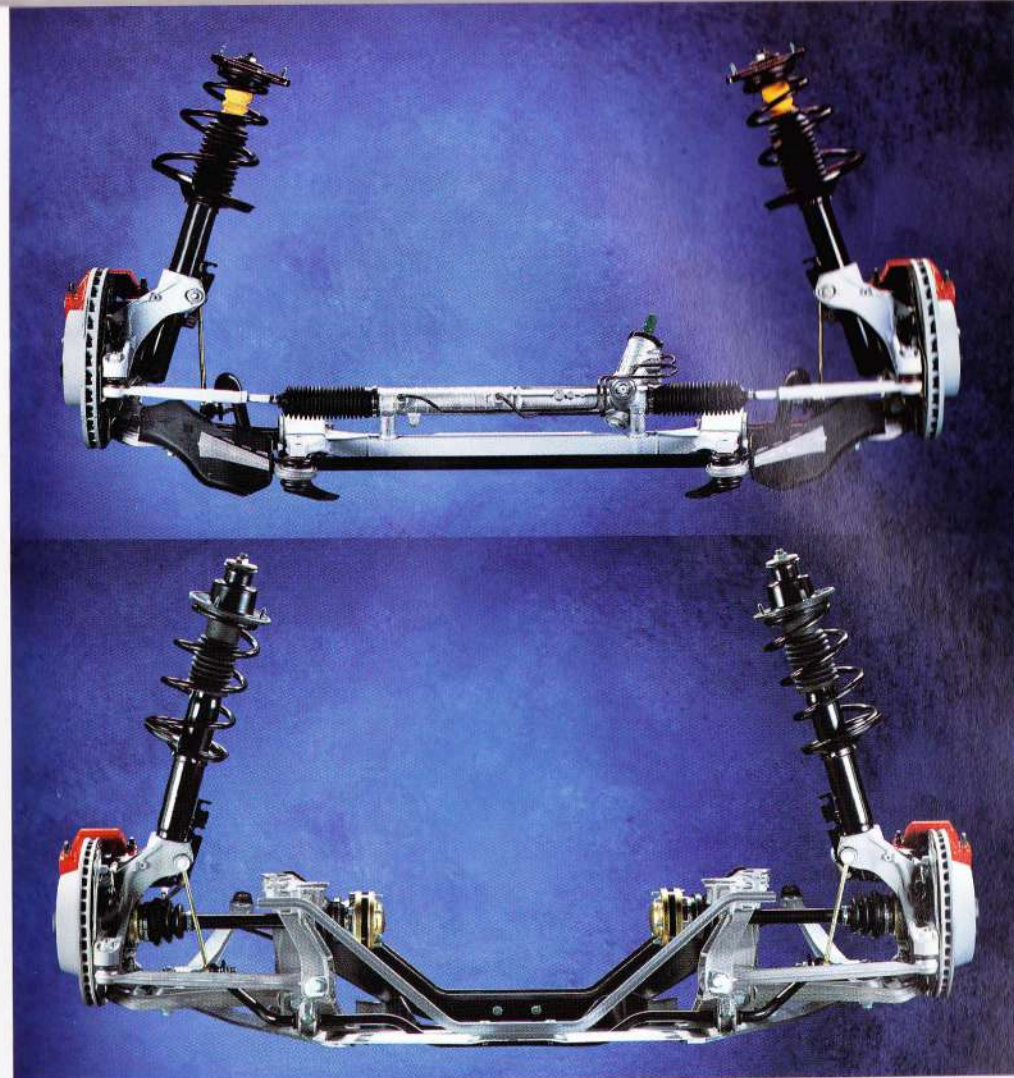
Essieu McPherson avec bras de suspension, jambe de force et étriers de freins rouges sur le Boxster S
